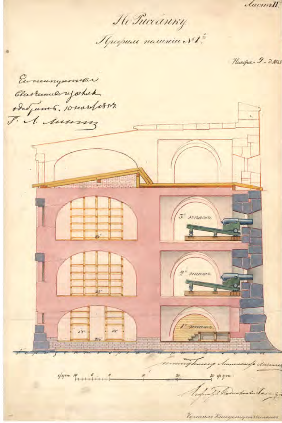
Проектный чертеж размещения орудий на трех этажах форта
